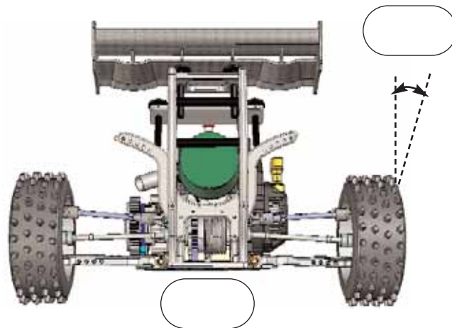
Bodenfreiheit und Sturz hinten ride height and camber rear
