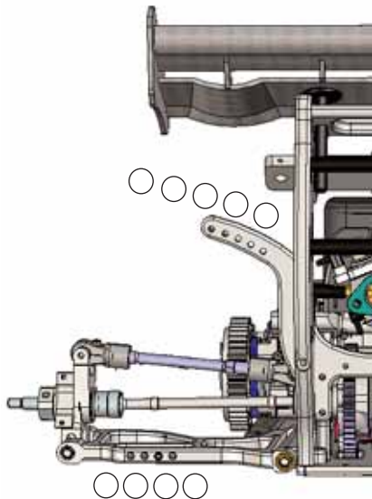
Dämpferposition hinten damper position rear
